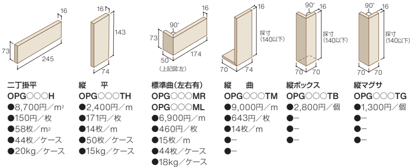
マガリ形状
