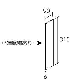
90×315mm平役物 受 ROM-LMG(ROM-TMSG用役物) ROM-LML(ROM-TMSL用役物) ROM-LGO(ROM-TGSO用役物) ROM-LGS(ROM-TGSS用役物) ●90×315×6mm 設計価格:6,800円／枚
